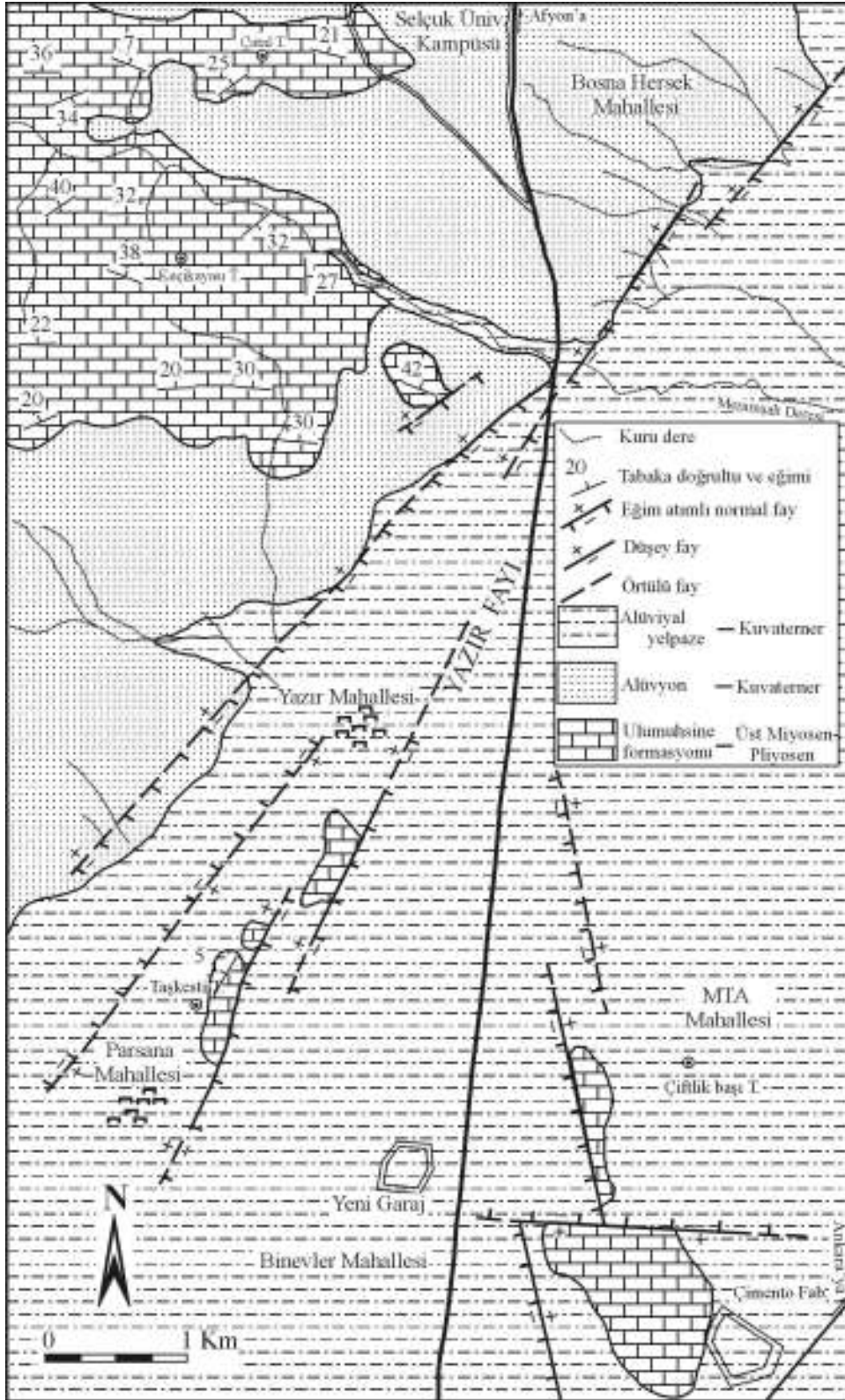
Şekil 2: İnceleme alanının jeoloji haritası
