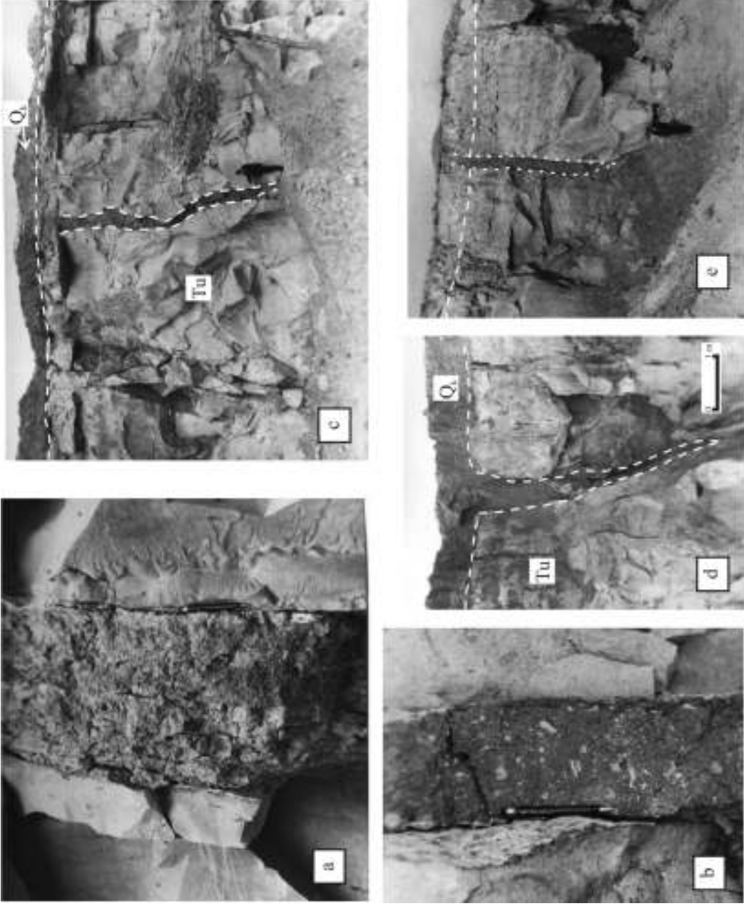
Levha 3: a, b: Kireçtaşlarında içi allüvyial çökeltilerle doldurulmuş yarıkların yakından görünüşü, c: Masif gölsel kireçtaşları içinde oluşan ve üstü tabakalı kireçtaşı ile örtülmüş bir yarık, d ve e: Gölsel kireçtaşlarını (Tu) tümden kesen ve üstteki Koriya formasyonu (Qk) içine kadar devam eden içi allüvyonla doldurulmuş yarıklar.
