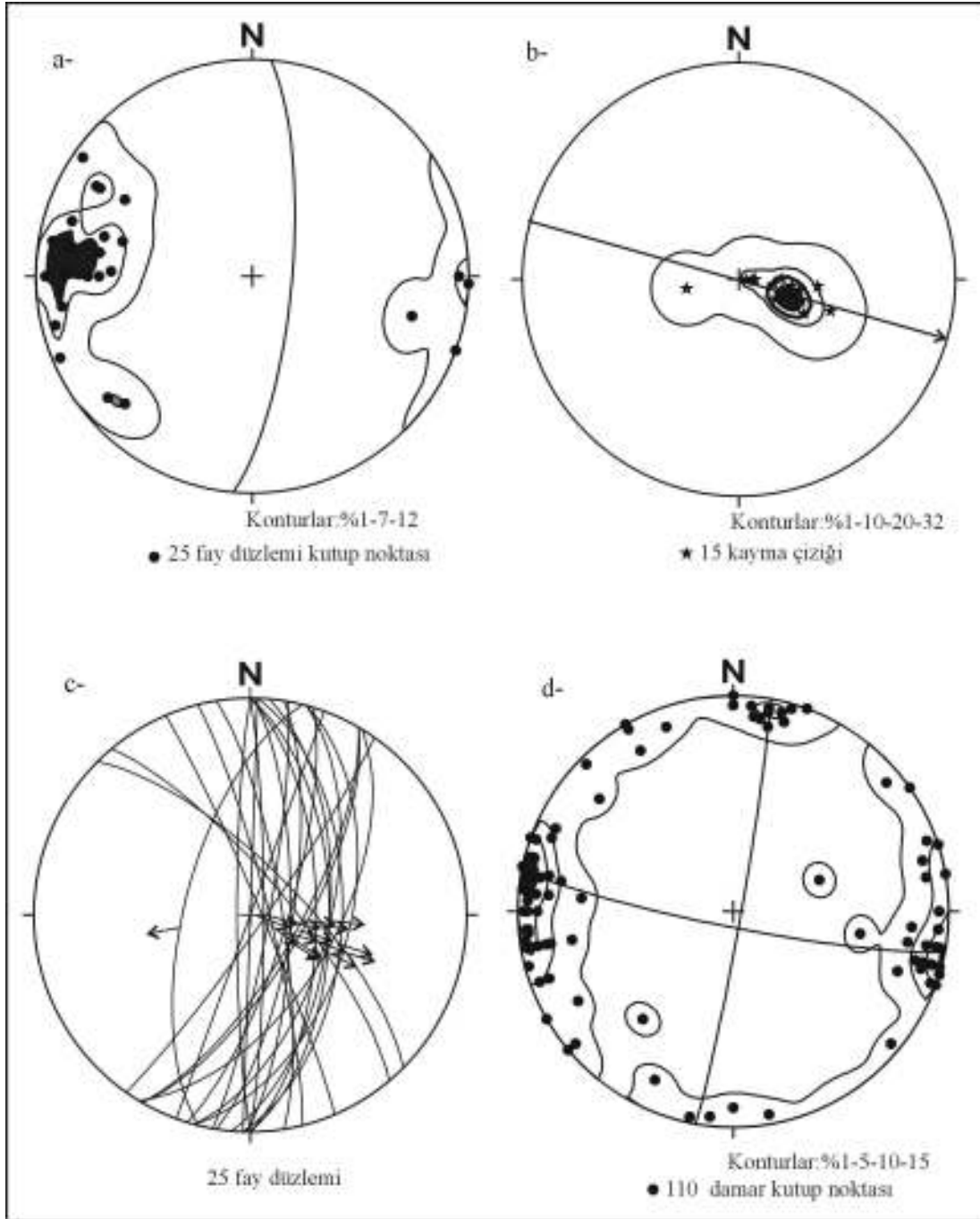
Şekil 3: a-Yazır fayına ait fay düzlemlerine ilişkin nokta-kontur diyagramı, b- Fay düzlemleri üzerinde ölçülmüş kayma çiziklerine ilişkin nokta-kontur diyagramı, c- Fay yüzeyleri ile kayma çiziklerini gösteren diyagram, d- Yazır ve Parsana Mahalleleri arasındaki taş ocaklarında ölçülmüş yarıklara ilişkin nokta-kontur diyagramı.
